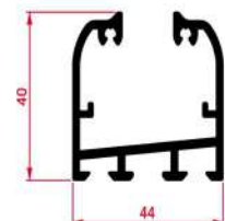
PERFIL MARCO INFERIOR | PROFIL CADRE INFERIEUR | SILL
