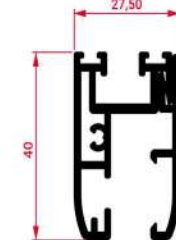
PERFIL HOJA EMBELLECEDOR | PROFIL VANTAUX COUVRE VIS | FRAME TRIM
